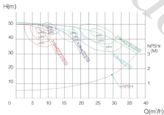
KS-30(Q-H曲线图) KS-30(Q-H curve)
