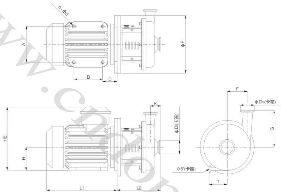
KS泵安装数据表(无罩)
